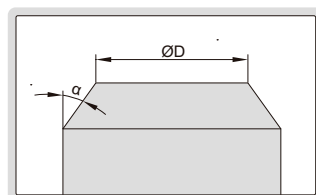
测量圆柱倒角的口端直径
